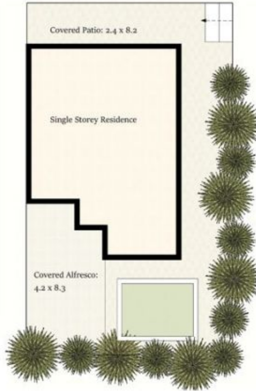
Site Plan:
